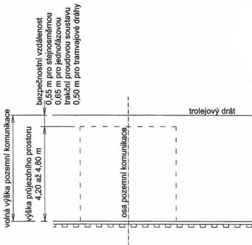
Obrázek 2 - Volná výška nad přejezdovou vozovkou
