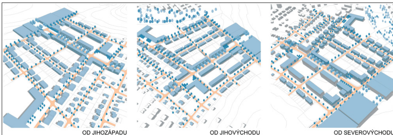
Obr. 5: Hmotový 3D model ověřující mantinely navržené prostorové regulace v rámci návrhu regulačního plánu Mlčovice-Mladá (autorka Victoria Cheremnykh, studentka Modulu PrP, letní semestr 2021/2022, vedoucí ateliéru Veronika Šindlerová)
