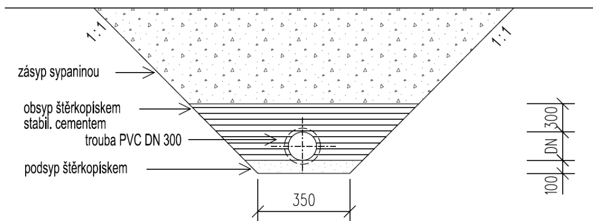
PŘÍČNÝ ŘEZ
