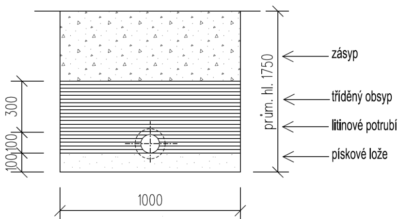
PŘÍČNÝ ŘEZ
