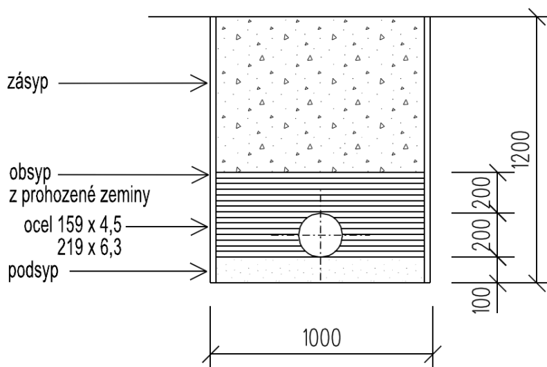
PŘÍČNÝ ŘEZ
