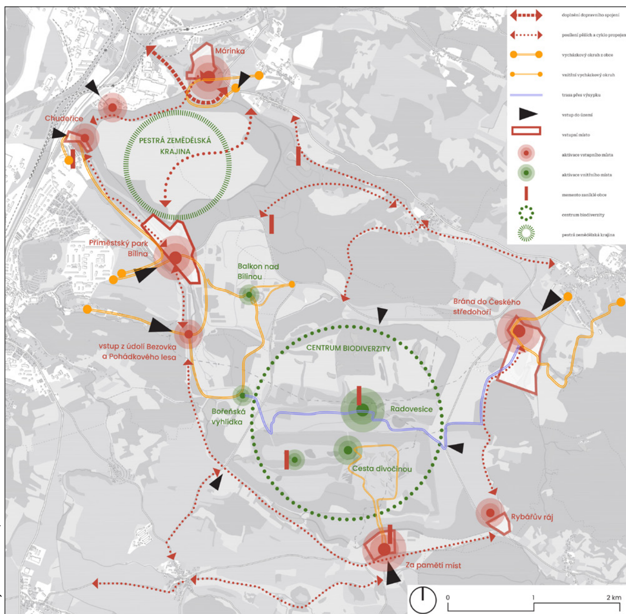
Obr. 7: Schéma koncepce rozvoje Radovesické výsypky
