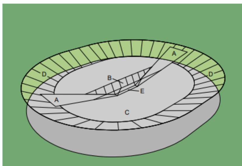
Ochranná pásma s výškovým omezením staveb pro nepřístrojovou RWY Letecký předpis L 14 – Letiště
