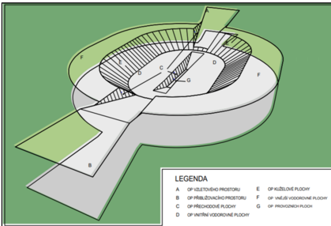
Obr. 36: Ochranná pásma vzletové a přistávací dráhy
