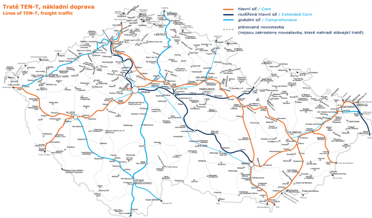
Obr. 33: Tratě mezinárodní nákladní dopravy TEN-T podle významu pro zavedení opatření a doby realizace
