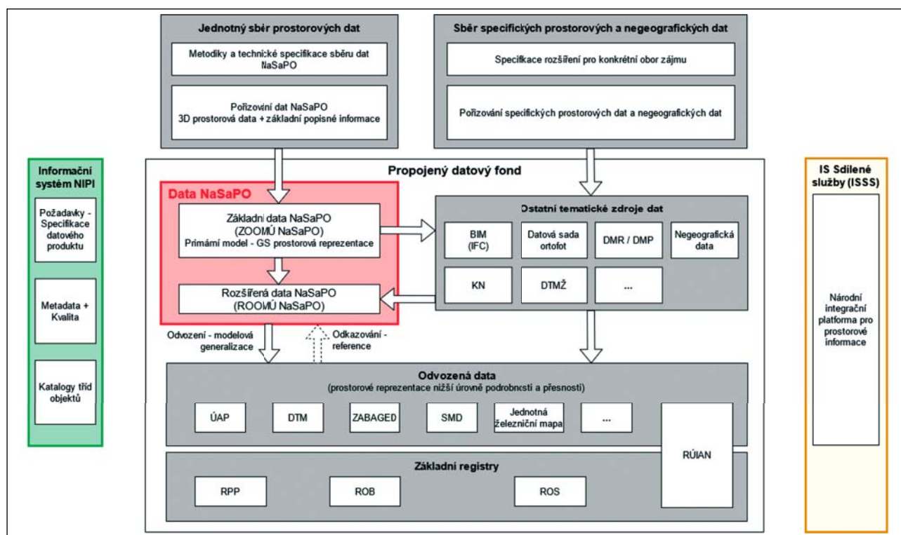
Toky dat do NaSaPO v propojeném datovém fondu, IS NIPI a ISSS
